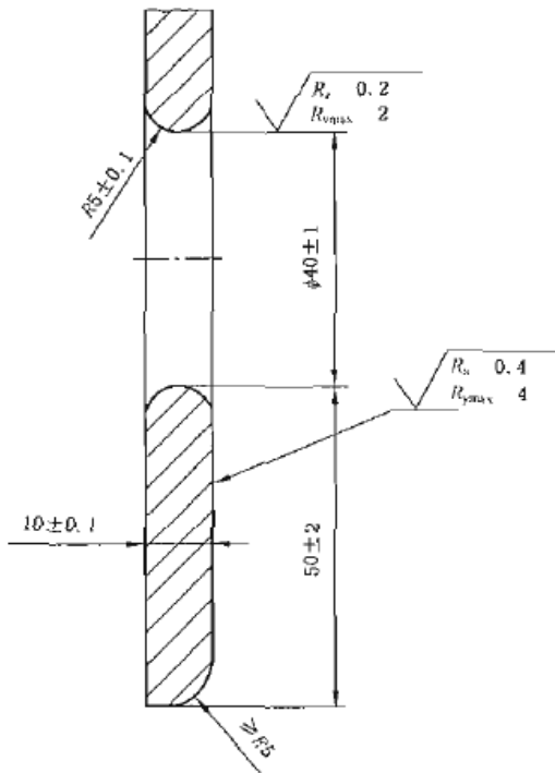
图 10 孔板示意图
