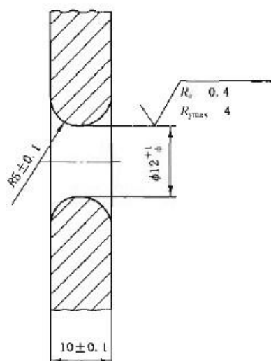
图6 孔板内孔质量要求
