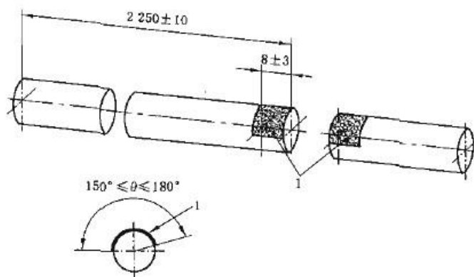
图5 护套滑移测试试样切割示意图
